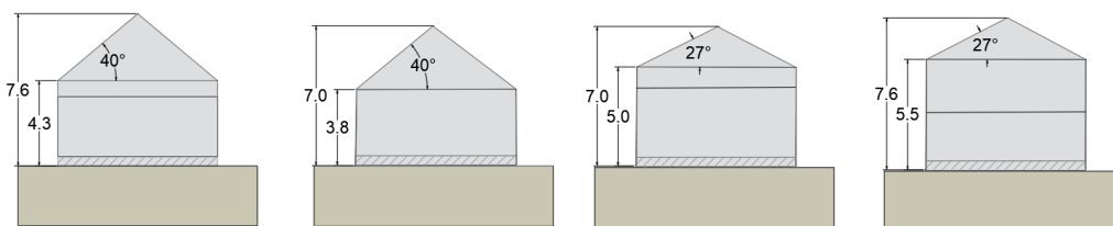
Illustration. Nockhöjd och takvinkel (Tyréns AB).
